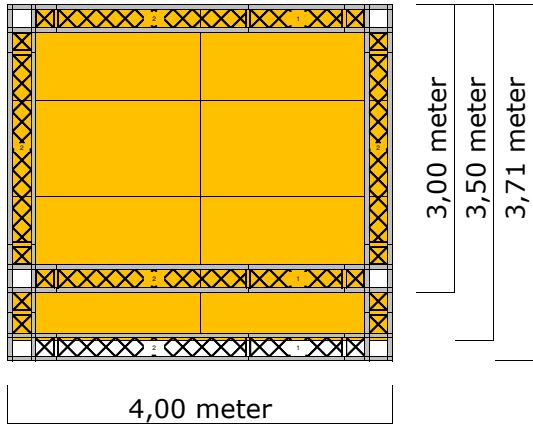
Boven aanzicht
