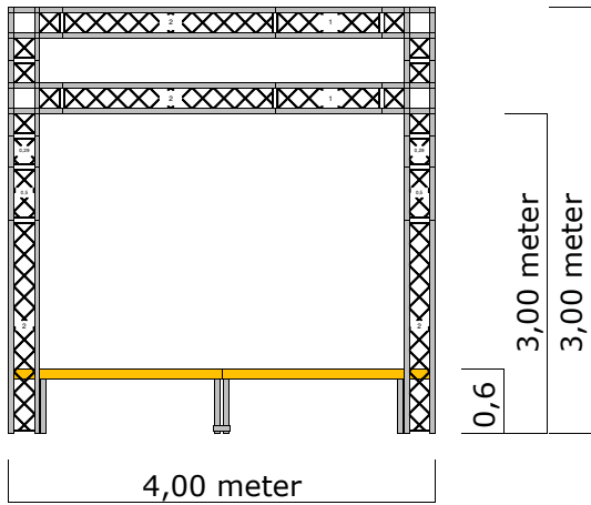
Voor aanzicht
