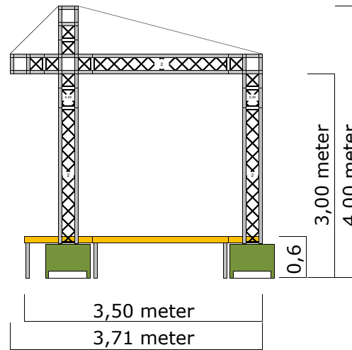
Zij aanzicht
